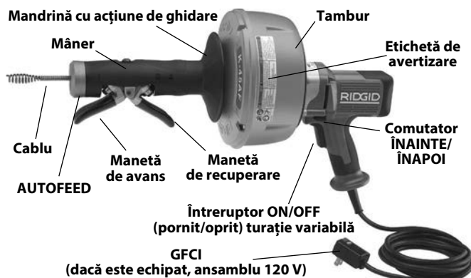
Figura 2 – K-45 AF Mașina de desfundat canale cu AUTOFEED (avans automat)
