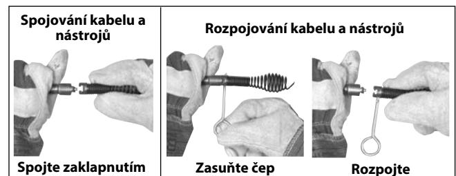
Obrázek 7 – Připojení a odpojení nástrojů
