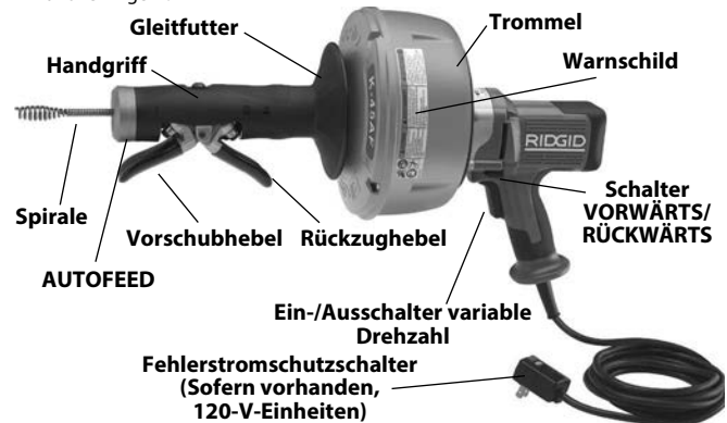
Abbildung 2 – K-45 AF Abflussreinigungsmaschine mit AUTOFEED
