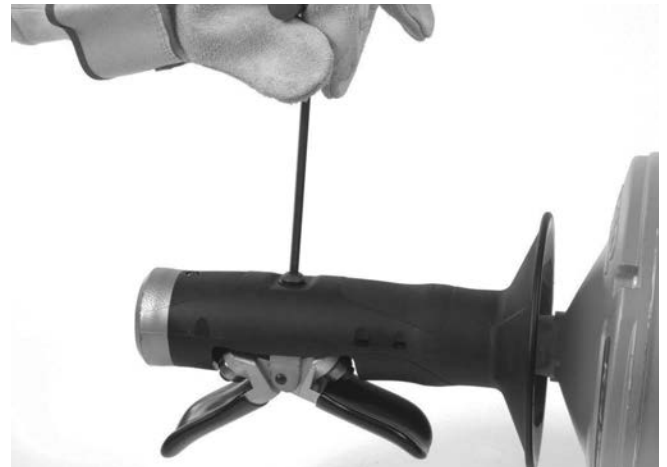
Εικόνα 12Α – Αφαίρεση βίδας μηχανισμού AUTOFEED
