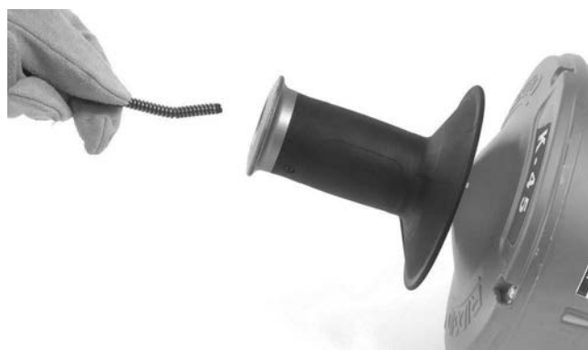
Figura 17 – Încărcarea cablului fără schimbarea tamburului interior
