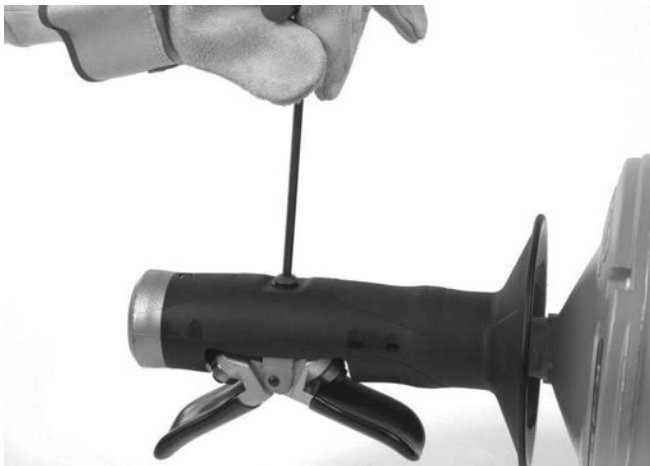
12А-сурет – AUTOFEED (АВТОМАТТЫ БЕРУ) бұрандасын шешу
